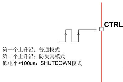
图7 软件设置 NS4158 工作模式
