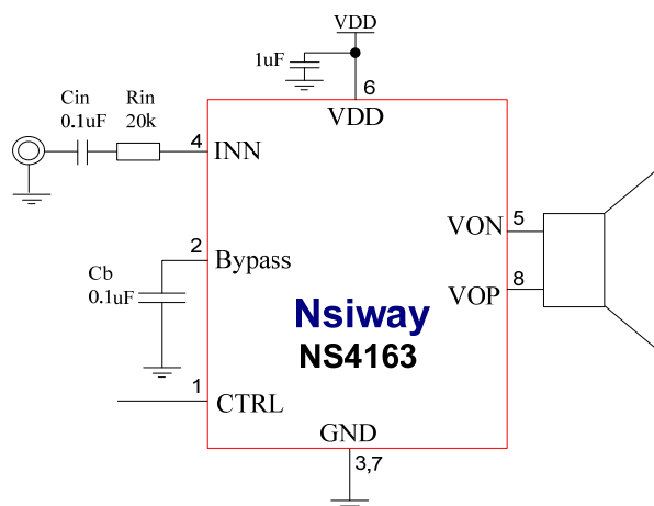
图1 NS4163 典型应用电路
