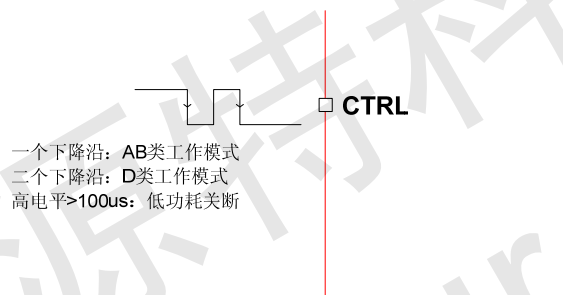
图4 NS4163 工作模式设置
