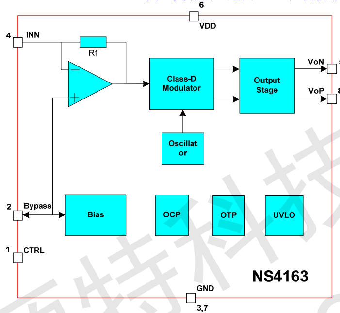
图3 NS4163 原理框图
