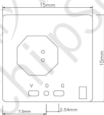
图 4.2 CST51L01-B 模块尺寸图 (引脚兼容 2.54mm 与 2.0mm 排针)
