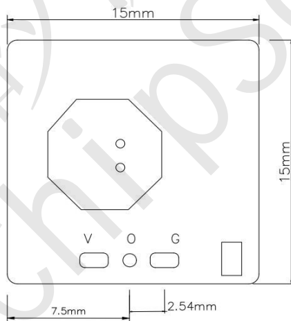
图 4.2 HY-RA10L15-B 模块尺寸图 (引脚兼容 2.54mm 与 2.0mm 排针)
